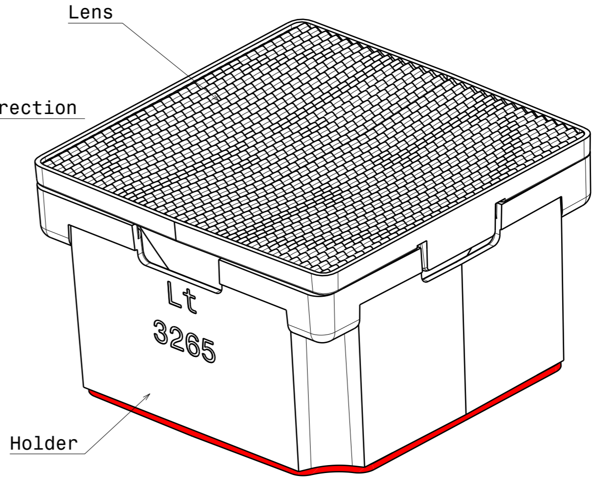
Isometric view Scale: 5:1
